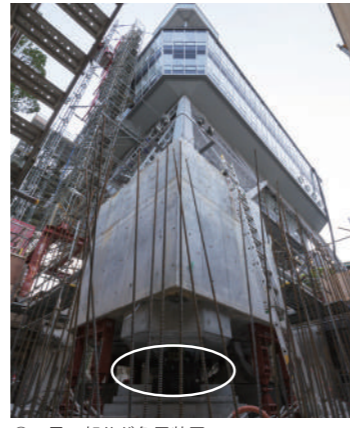
○の黒い部分が免震装置。ここで揺れを吸収します
